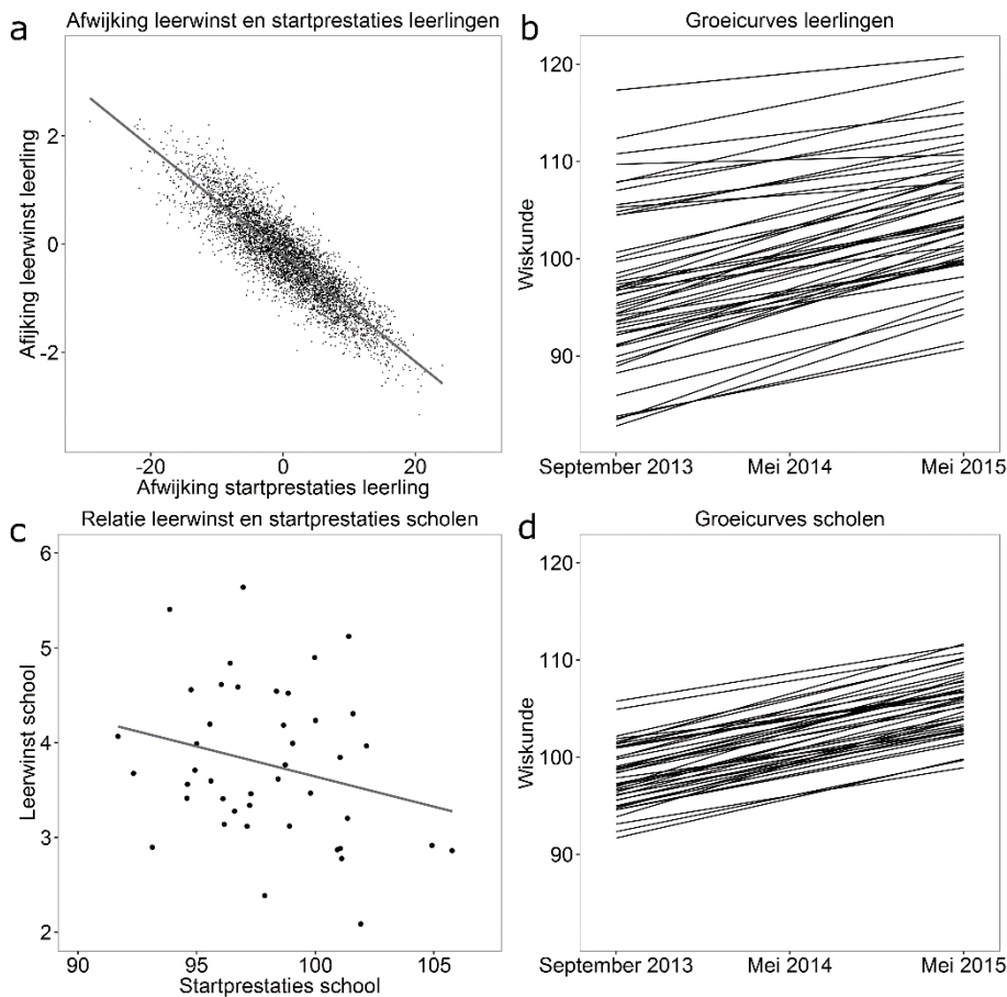
Figuur 1 Voorspelde groeicurves scholen model o
