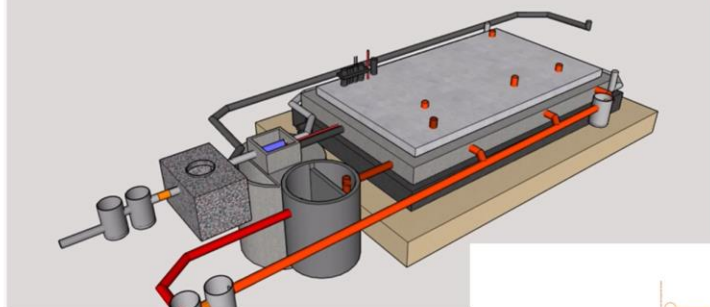
Funderings- en rioleringsopbouw met een gescheiden stelsel
